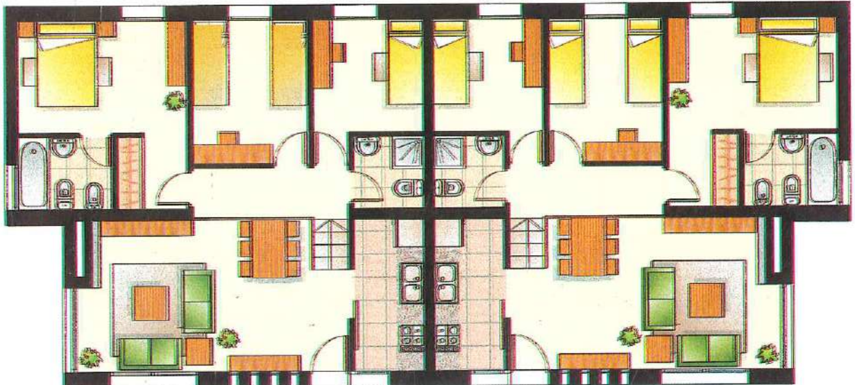
VIVIENDA TIPO B 3 DORMITORIOS Superficie construida = 76.51 m 2
